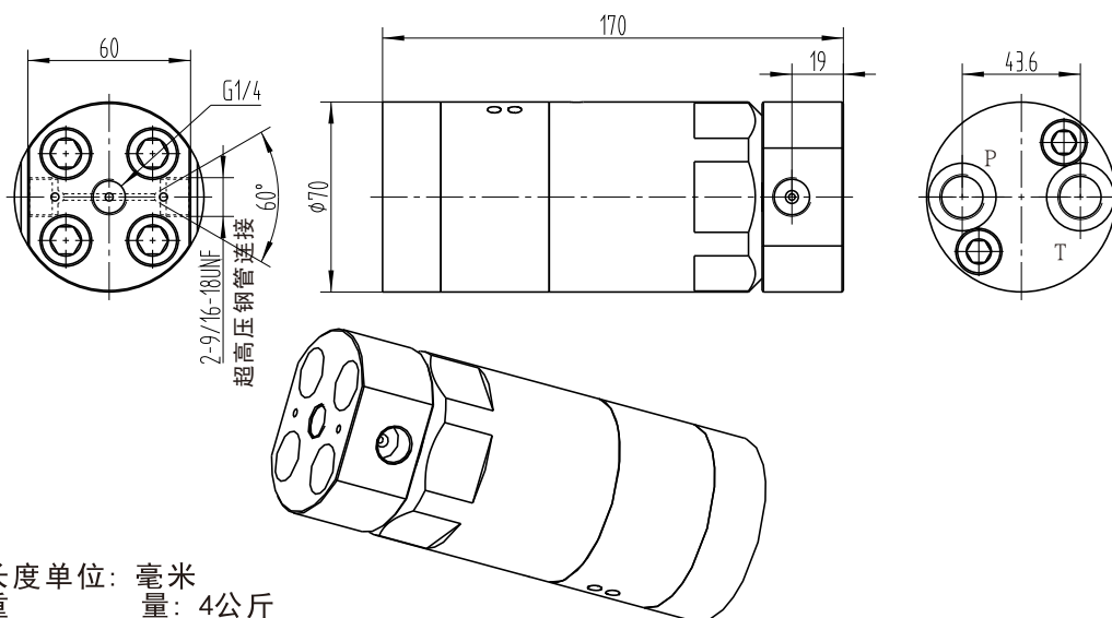
安装尺寸 Dimensions
