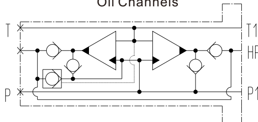
油路符号 Oil Channels
